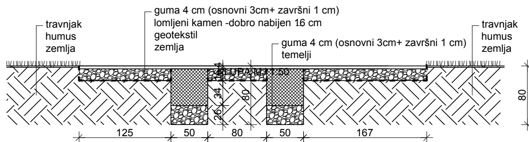
PRESJEK 1-1
